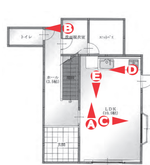
リフォーム前の平面図
